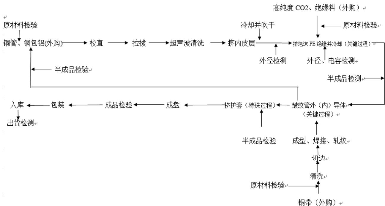
图1 馈线产品生产工艺流程图
